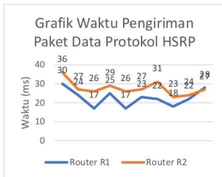
Gambar 11. Grafik Uji Coba Protokol HSRP
